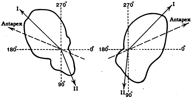
iv. Region VI. ; centre R.A. 16^{\text{h}} , Dec. +50^{\circ} .
